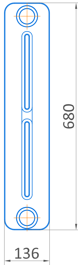
секция без ножек
